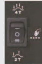
Зварювання в MIG режимі - 2, 4 такти та точкове зварювання
