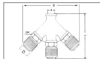
Розподільники трьохканальні. Внутрішня різьба
