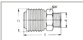
Зовнішня різьба
