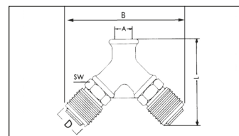
Розподільники двоканальні. Внутрішня різьба
