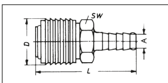
Шланговий з'єднувач
